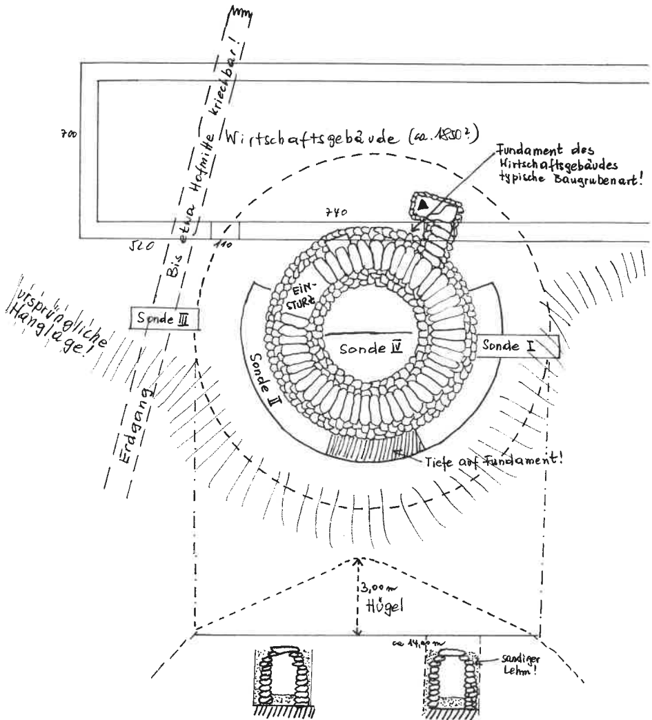
Rundbau in Puchegg 59, „Haas in Kerschbaumhof“.
