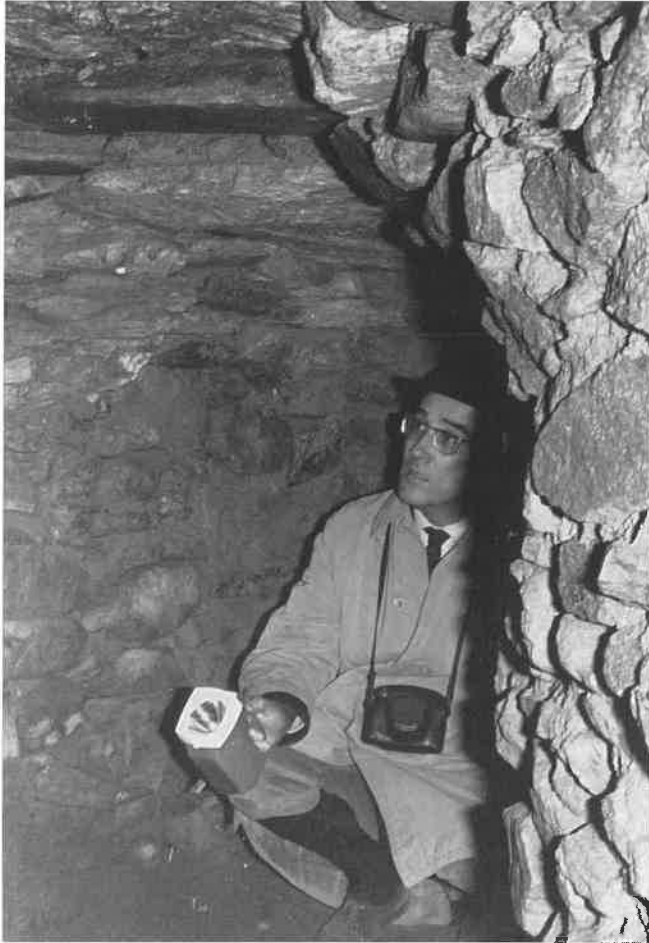
Univ.-Prof. Dr. H. Baltl, der Vorsitzende des Frühmittelalter-Ausschusses, im Inneren des Rundganges. Deutlich sind die Scheingewölbetechnik und die flachen Abdeckplatten zu erkennen.
